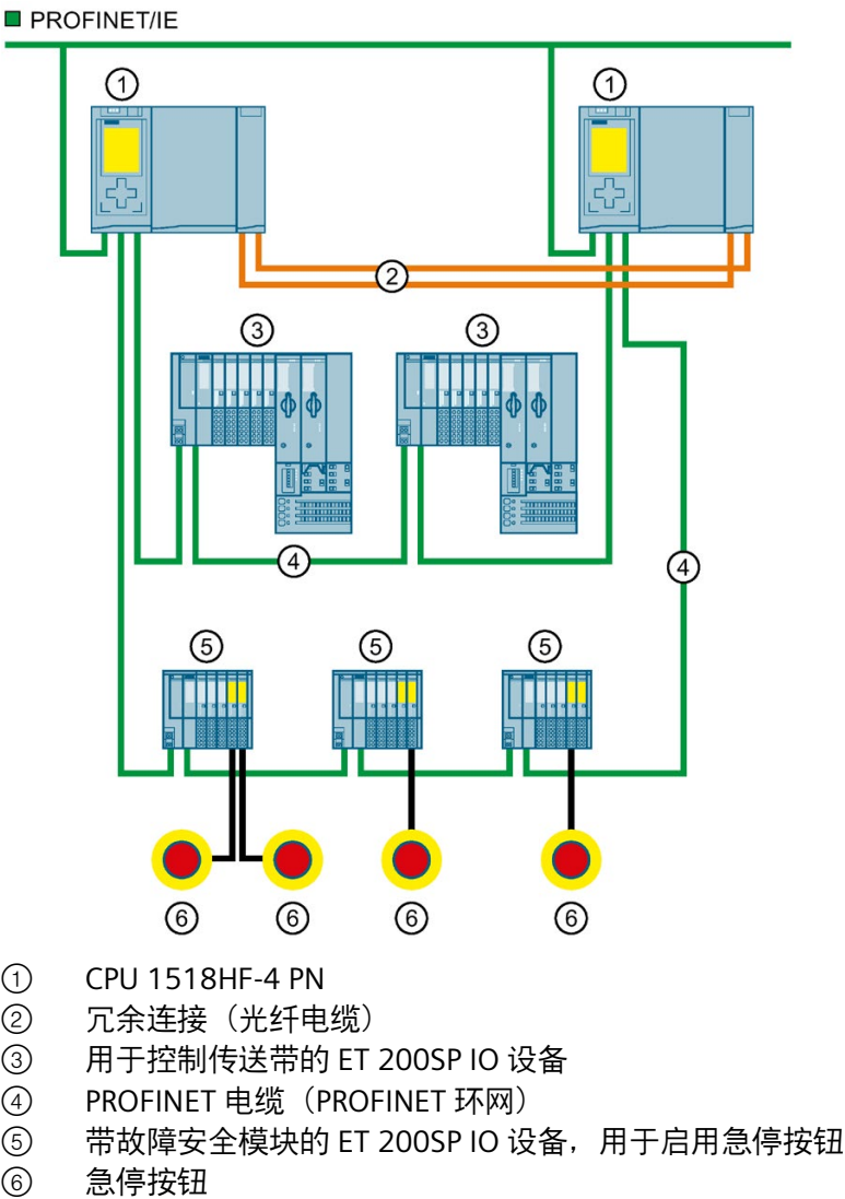
图 4-20 采用 CPU 1518HF-4 PN 和 ET 200SP 并带有故障安全模块的组态
