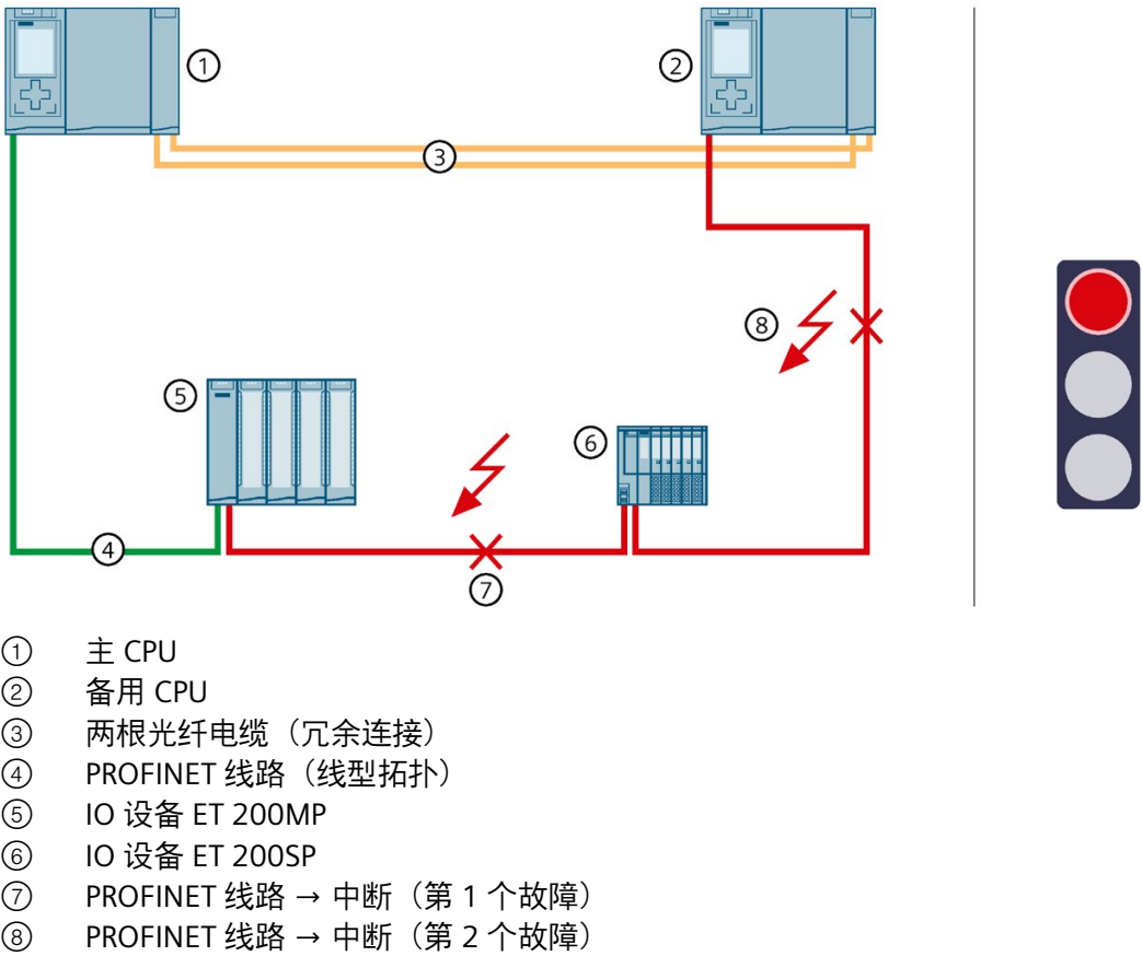
图 5-47 包含 S2 设备的线型拓扑中两个位置的 PROFINET 线路故障
