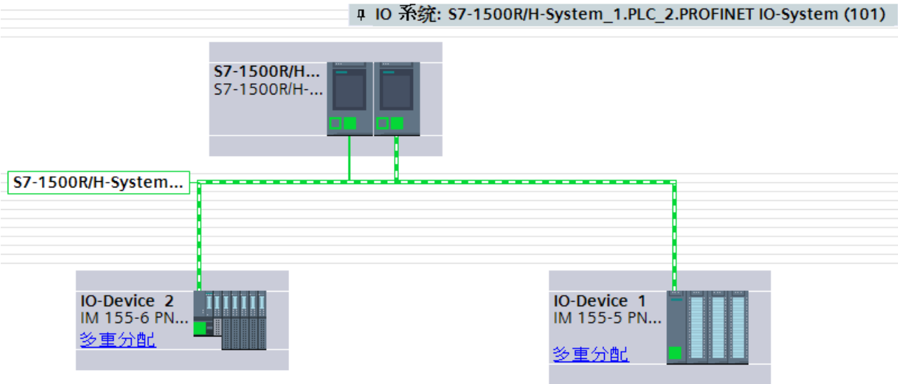
图 8-5 采用系统冗余的网络视图中分配的 IO 设备
