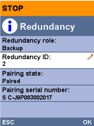
图 11-3 分配冗余 ID
