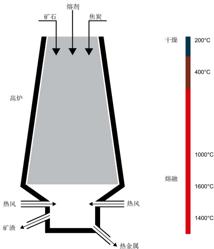
图 4-3 示例：高炉
