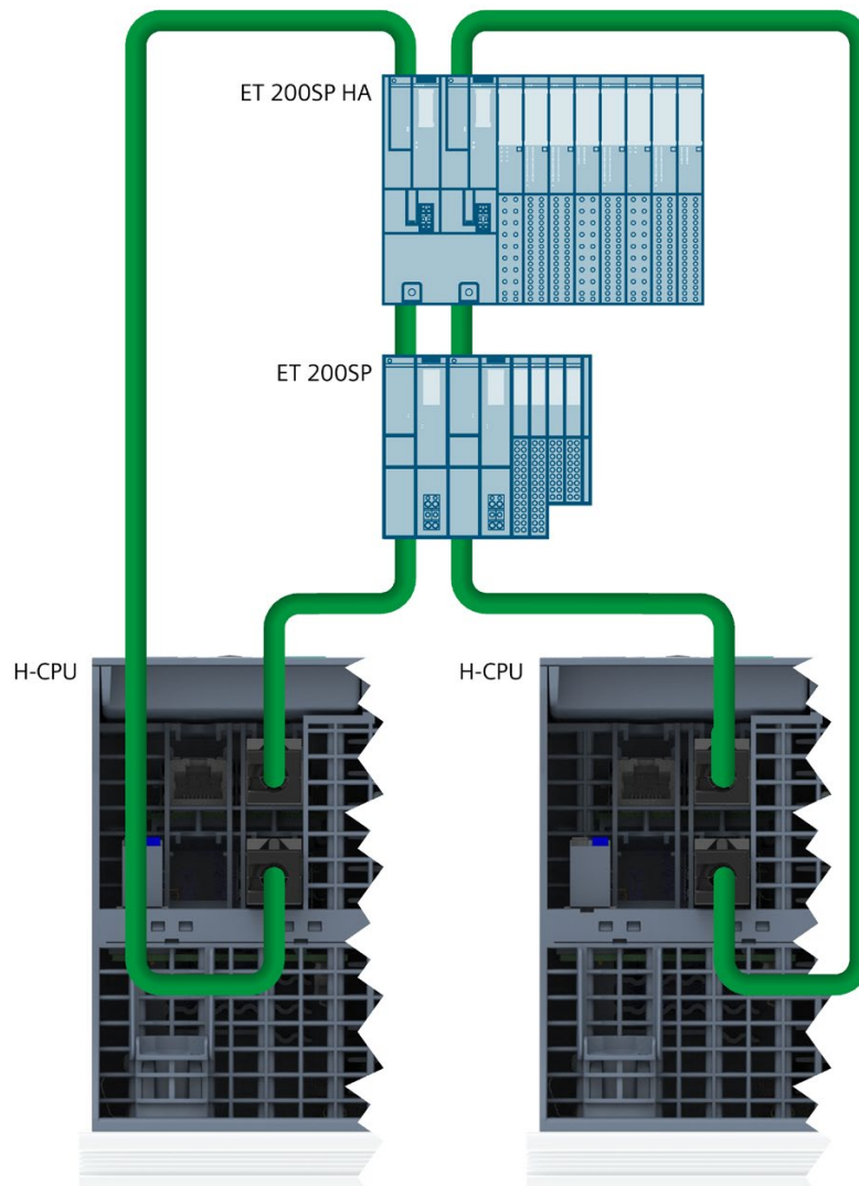
图 7-14 连接包含 R1 设备的 PROFINET 环网
