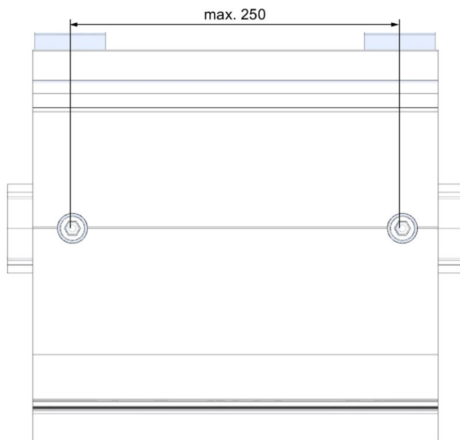
图 6-6 两个 DIN 导轨适配器之间的距离
