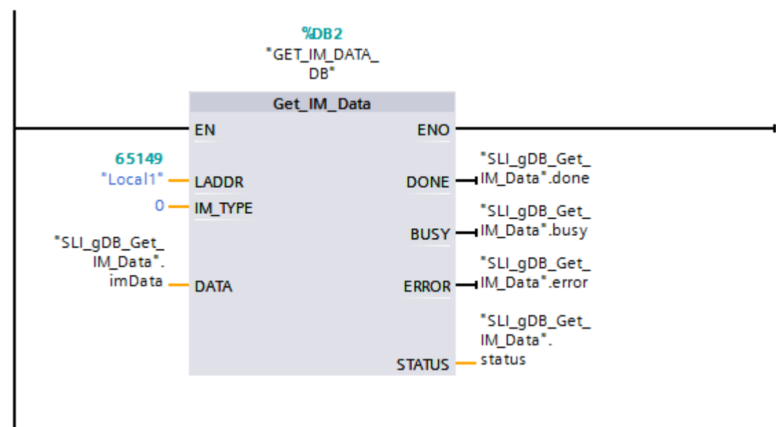
图 11-16 示例：从 S7-1500R 冗余系统读取 I&M0 数据
