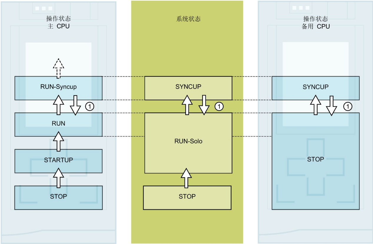
图 11-8 SYNCUP 系统状态中止
