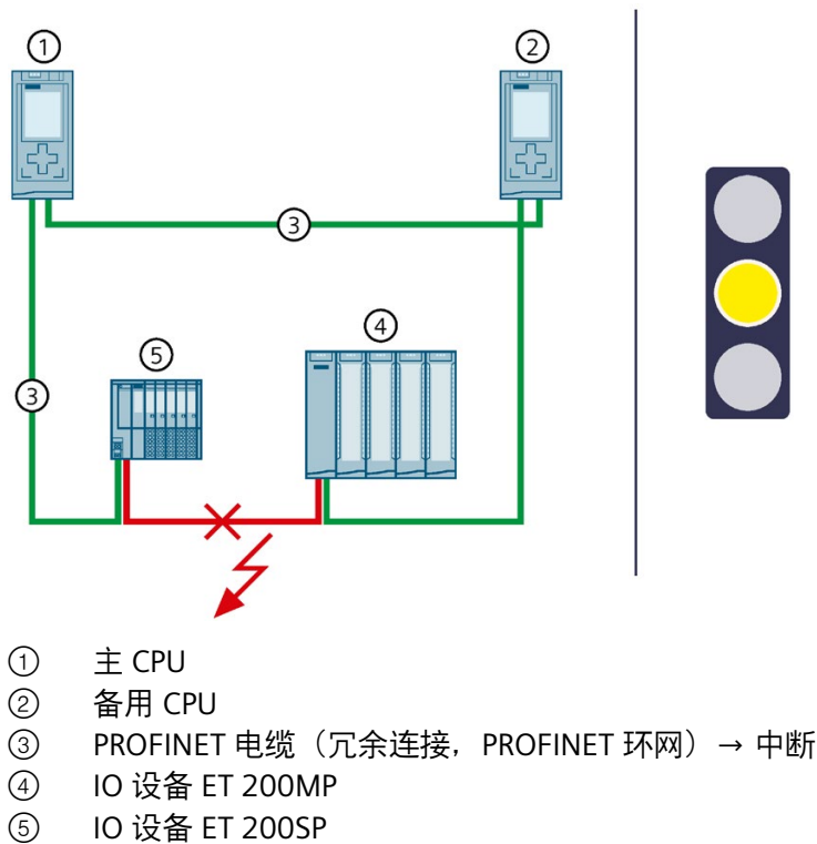
图 5-26 PROFINET 环网中的 PROFINET 电缆故障（以 S7-1500R 为例）
