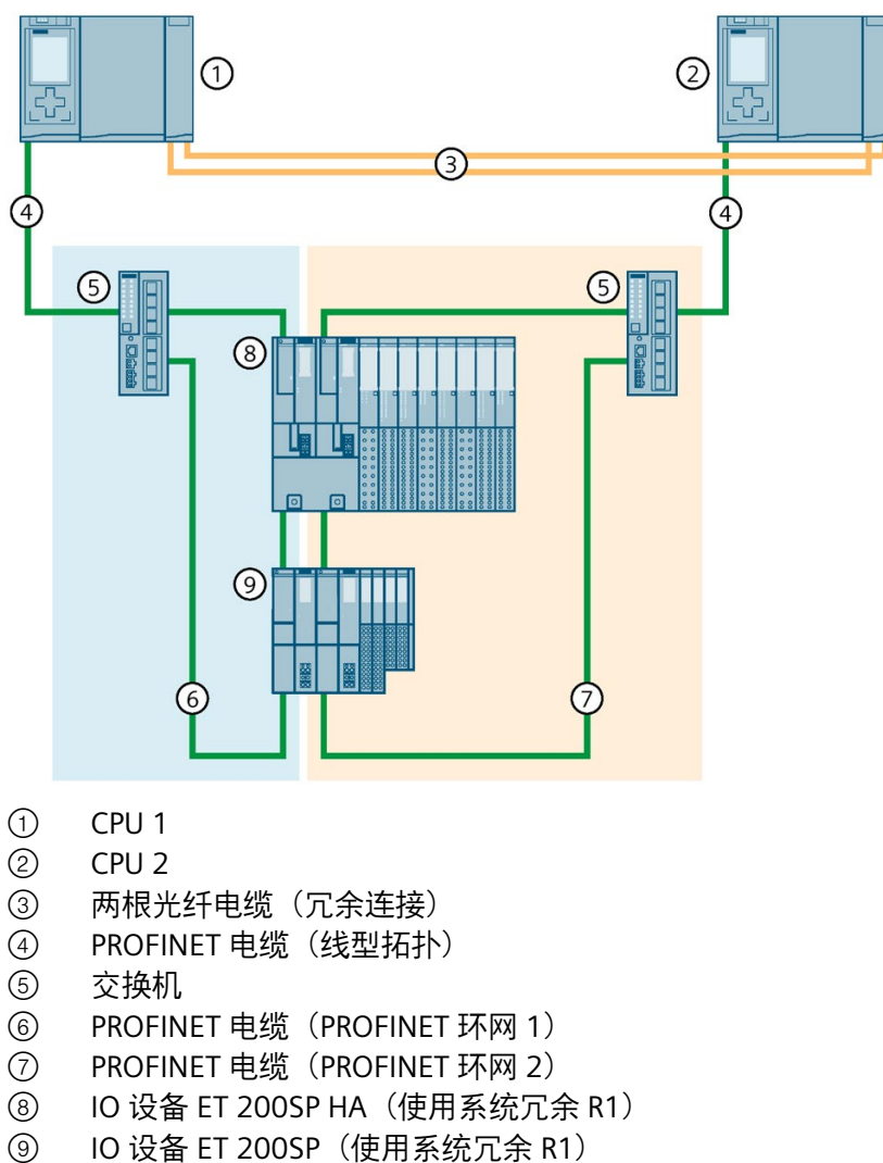
图 5-15 线型拓扑中包含 R1 设备和交换机的 S7-1500H 组态
