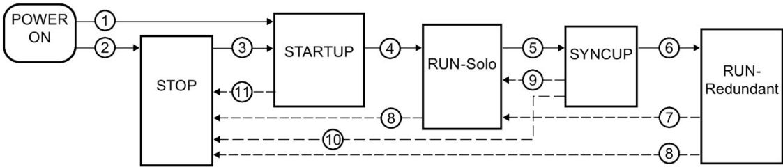
图 11-9 系统状态转换
