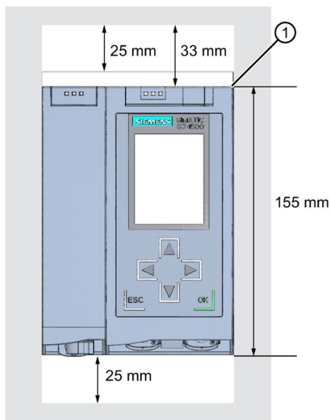
图 6-1 控制柜中的最小间隙
