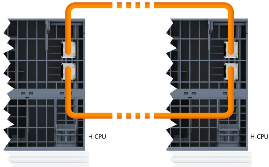
图 7-12 将冗余连接（光纤电缆）连接至 S7-1500H
