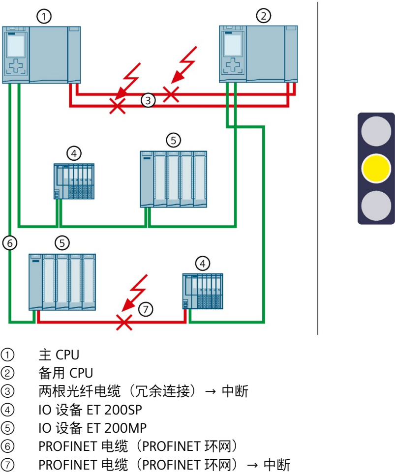
图 5-29 PROFINET 环网中的两个冗余连接和 PROFINET 电缆均发生故障
