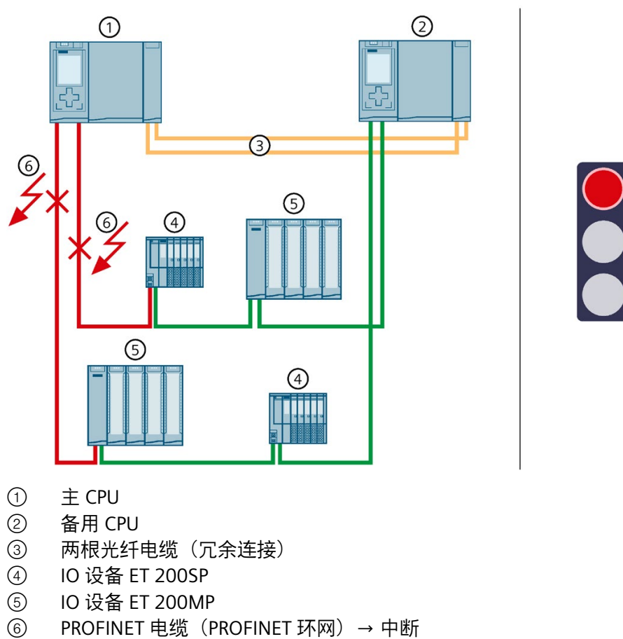
图 5-43 主 CPU 的 PROFINET 环网中的两根 PROFINET 电缆故障
