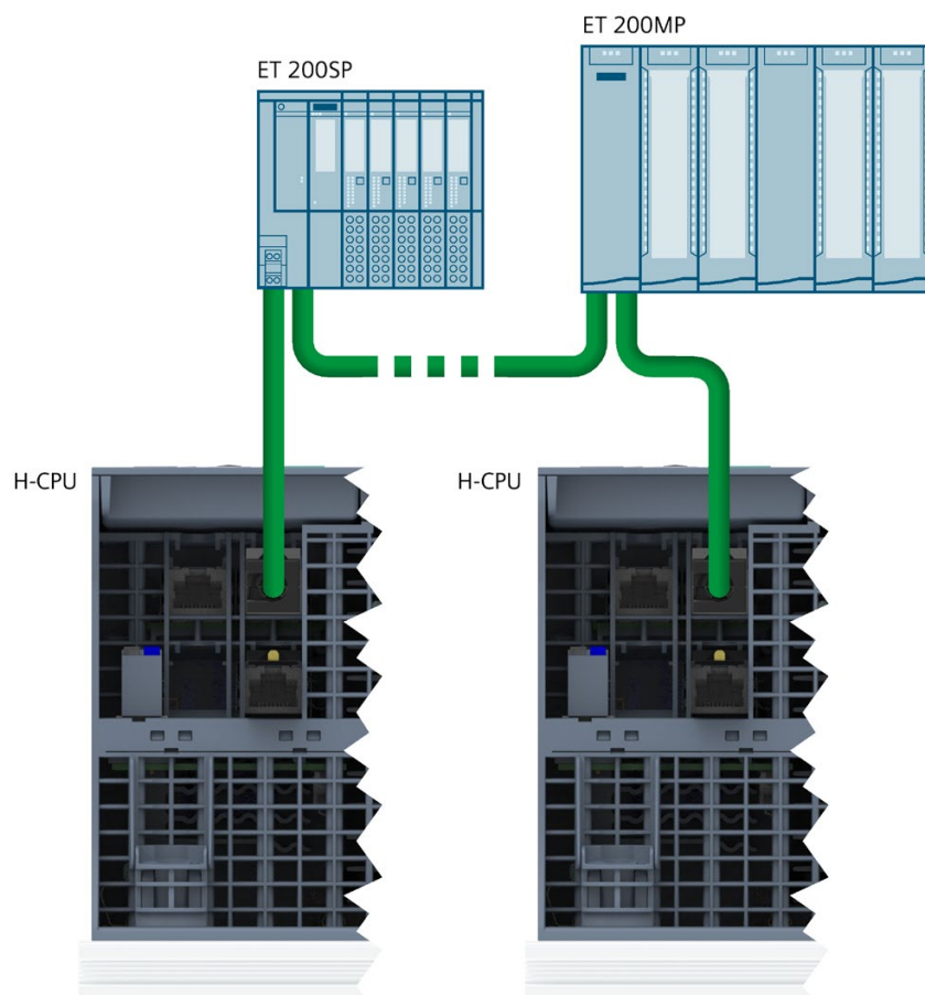
图 7-15 将包含 S2 设备的线型拓扑连接到 S7-1500H
