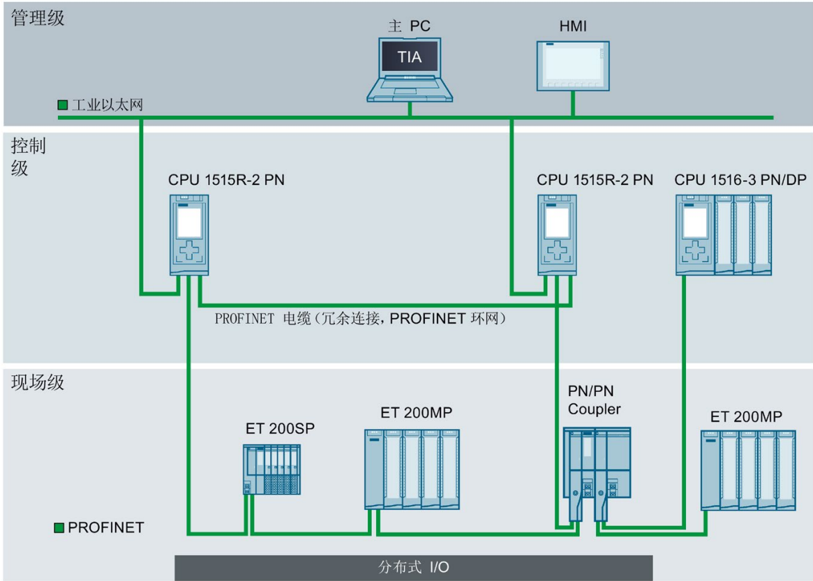
图 4-10 以 S7-1500R 为例介绍管理、控制和现场层级的可能组态
