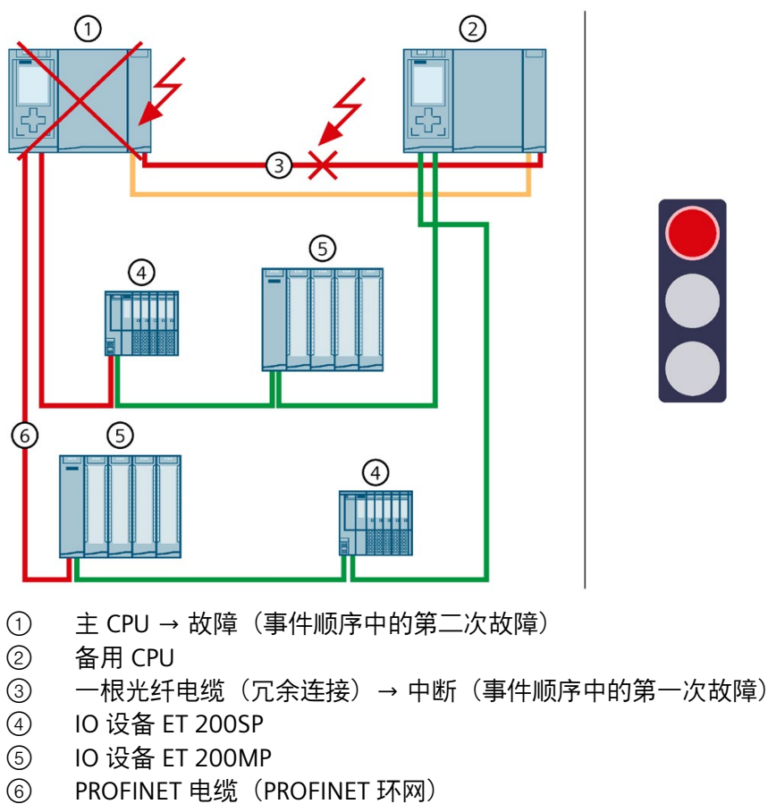
图 5-42 冗余连接和主 CPU 故障
