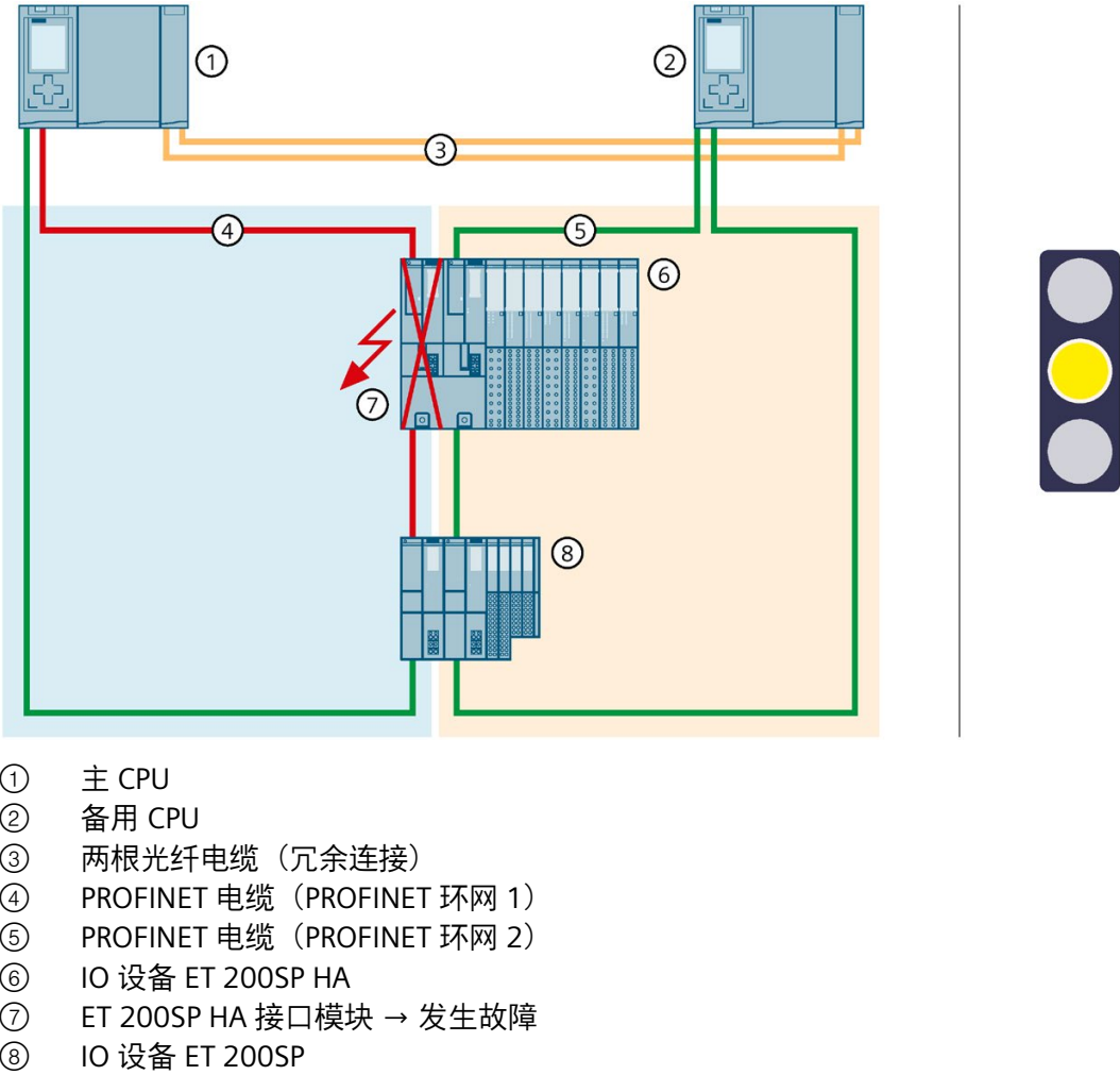
图 5-31 PROFINET 环网中 R1 设备中的接口模块故障
