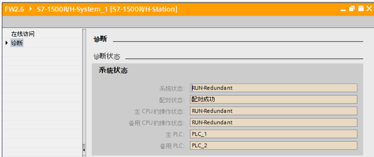
图 13-1 “已配对”诊断状态
