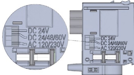
图 13-4 电源连接器上的标签
