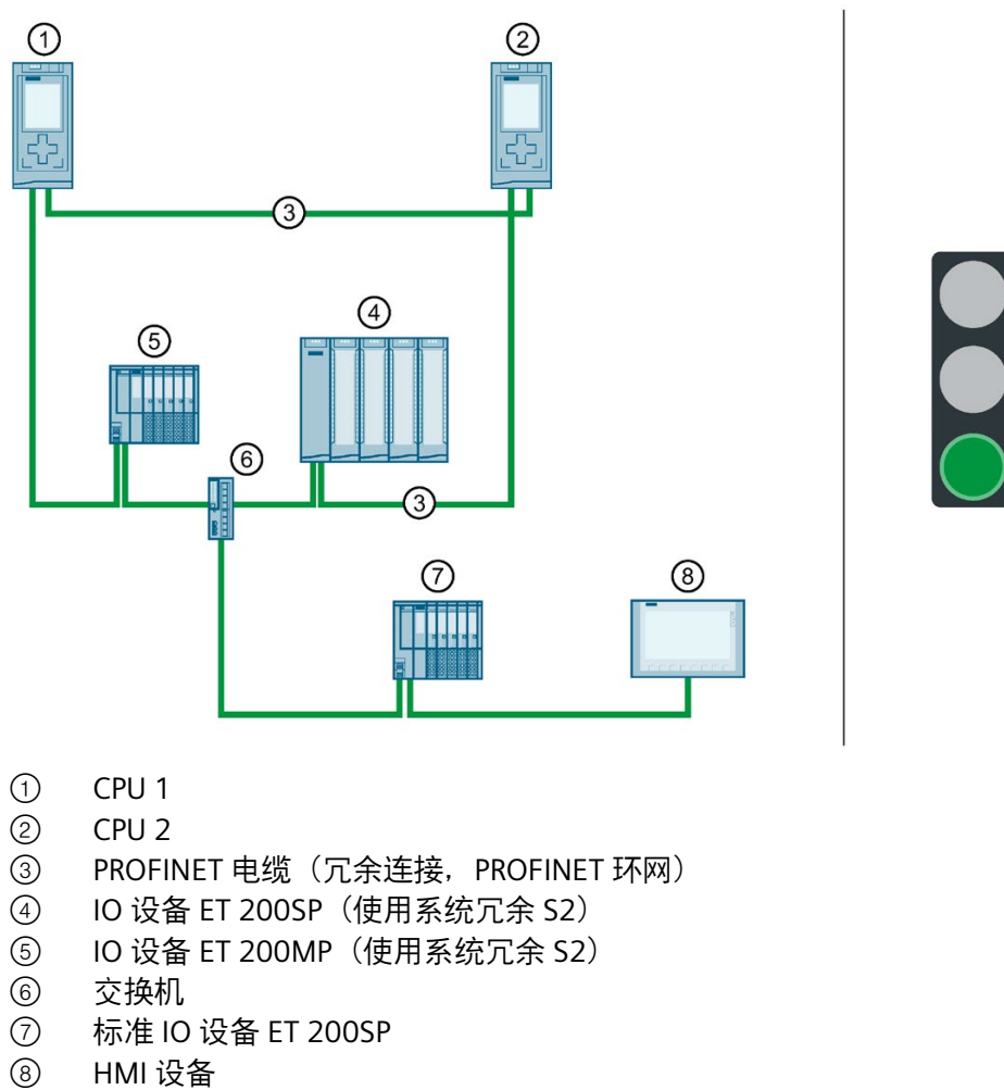
图 5-4 采用交换机和其它线型拓扑的 S7-1500R 组态
