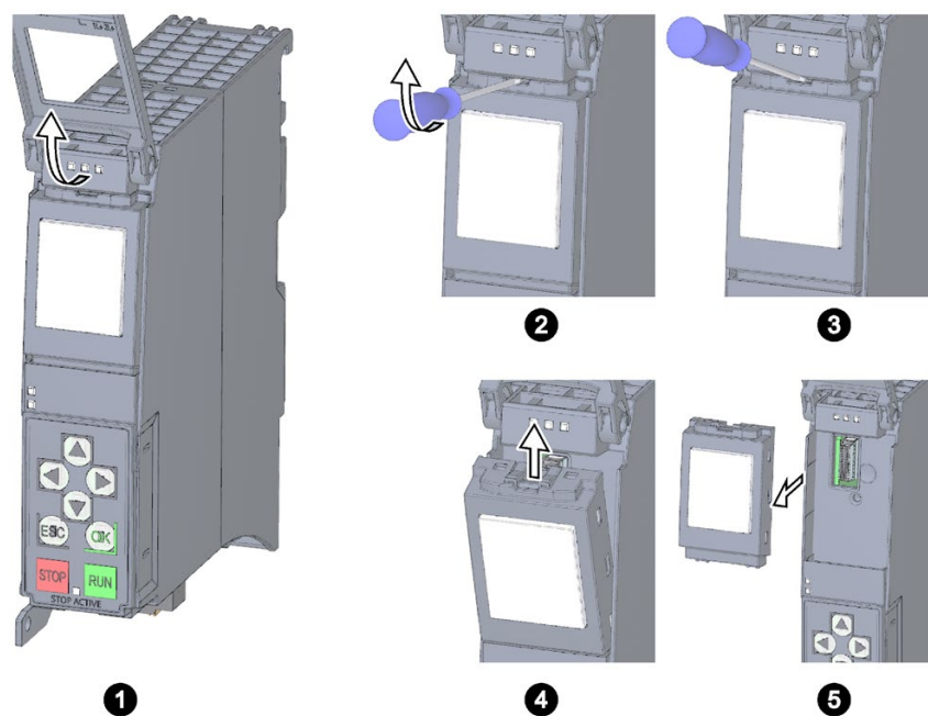
图 13-2 卸下显示屏
