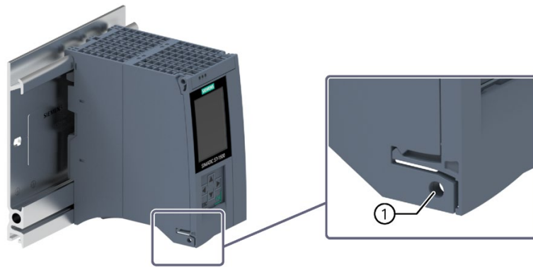
① CPU 上的锁紧装置
