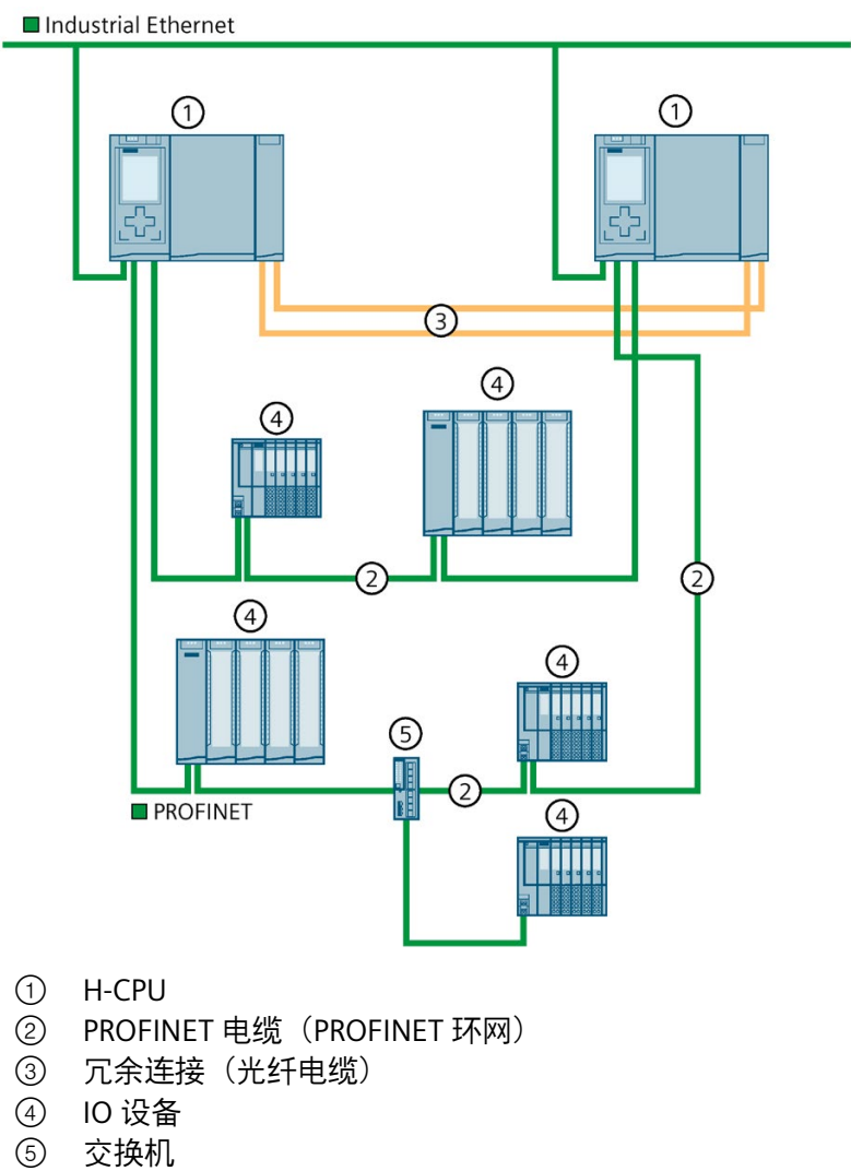
图 4-5 PROFINET 环网中连接了 IO 设备的 S7-1500H 组态
