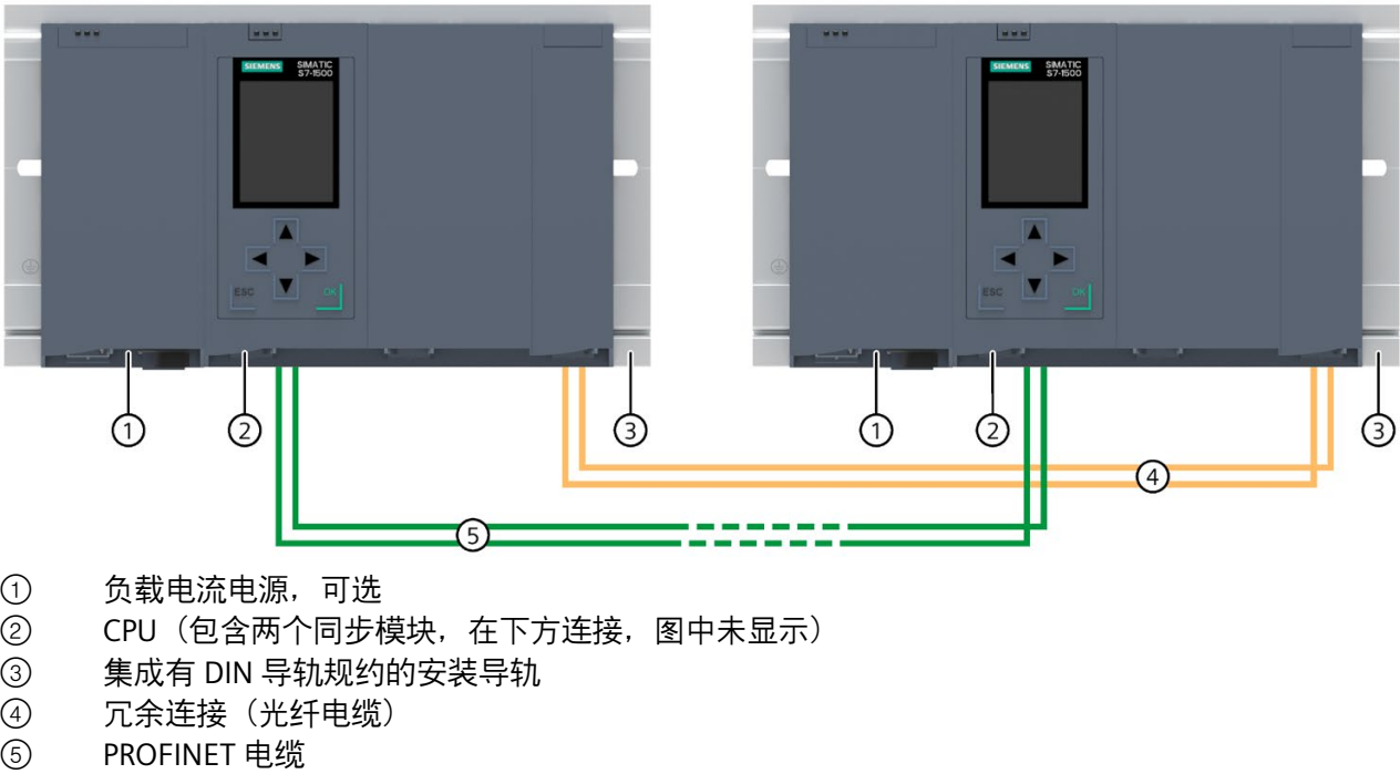
图 4-15 S7-1500H 组态示例
