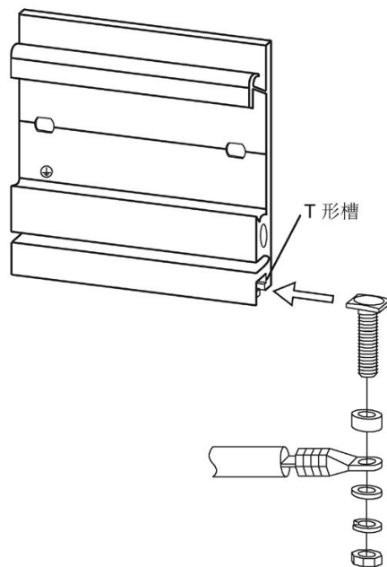
图 6-3 连接保护性导线（保护接地）
