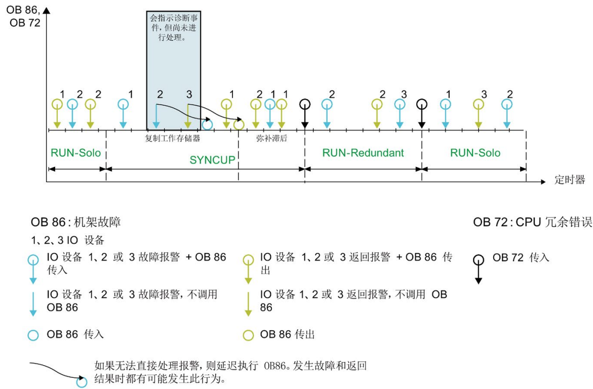
图 9-1 系统状态转换期间的 OB 72 和 OB 86
