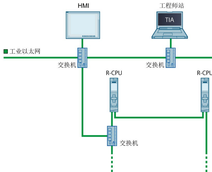
图 5-50 组态示例 CPU 1513R-1 PN：通过交换机连接 HMI 设备
