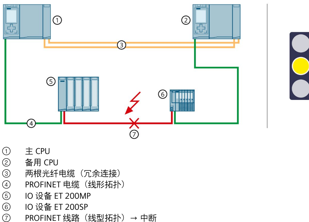
图 5-34 线型拓扑中两个 S2 设备之间的 PROFINET 线路故障
