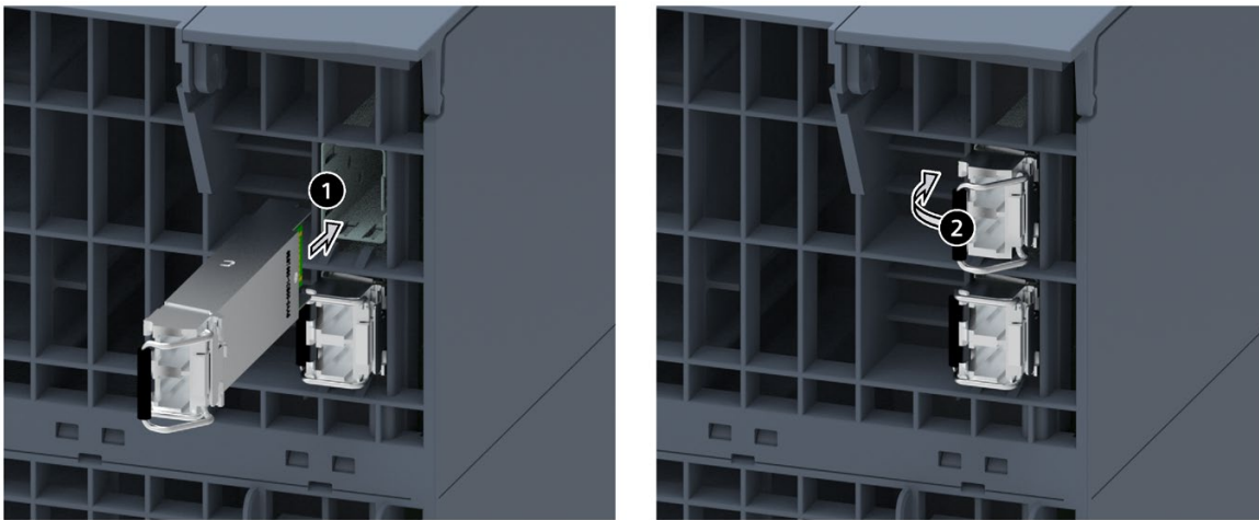
图 7-11 插入并锁定同步模块
