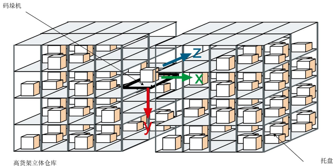
图 4-2 示例：高货架立体仓库
