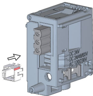
图 13-5 将编码元件插入电源连接器
