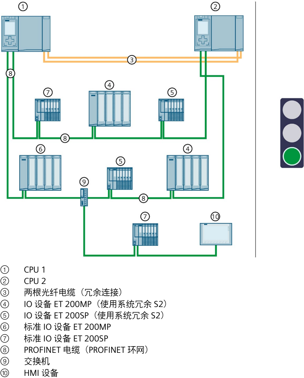
图 5-5 采用交换机和其它线型拓扑的 S7-1500H 组态
