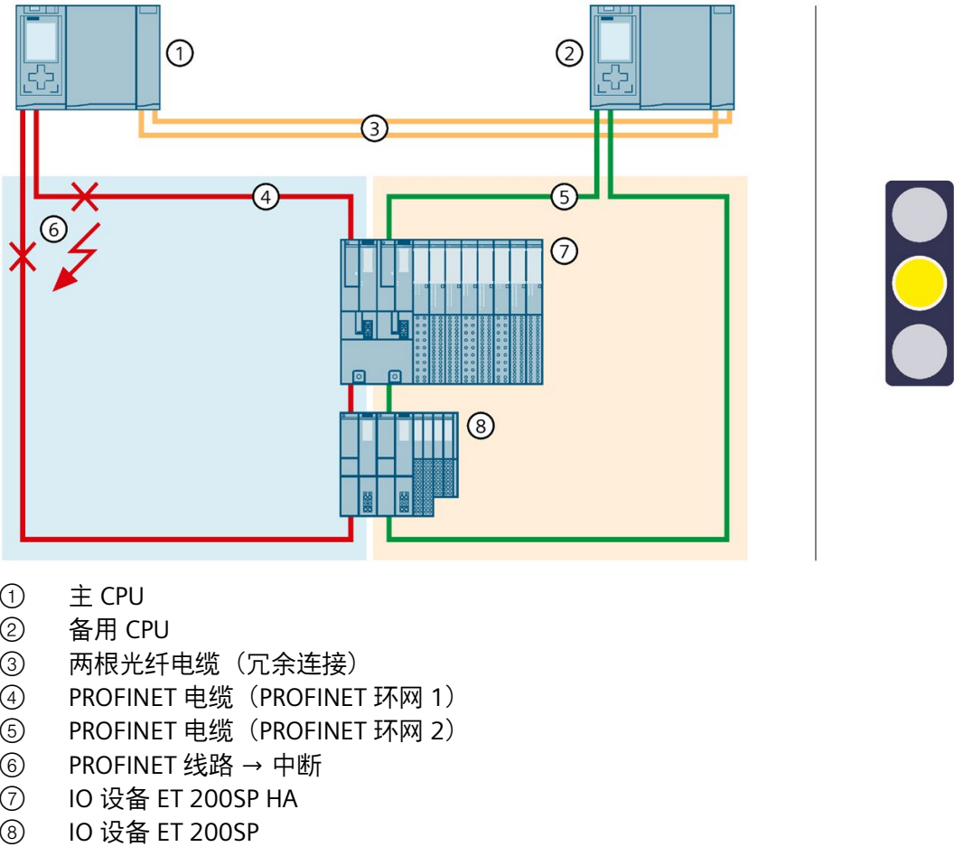
图 5-32 主 CPU 的 PROFINET 环网 1 中的两条 PROFINET 线路故障。
