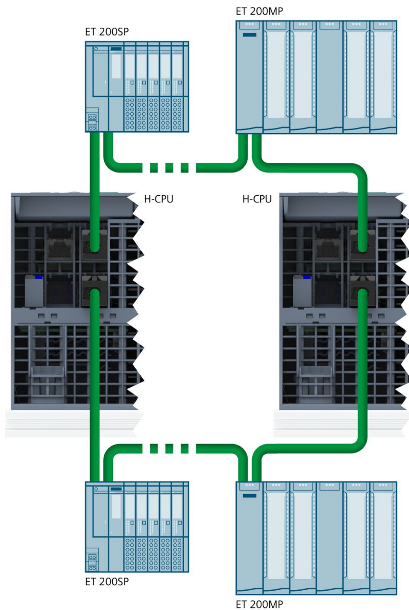
图 7-13 连接包含 S2 设备的 PROFINET 环网
