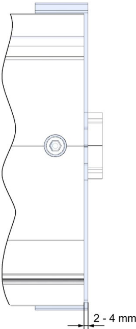
图 6-7 DIN 导轨适配器突出
