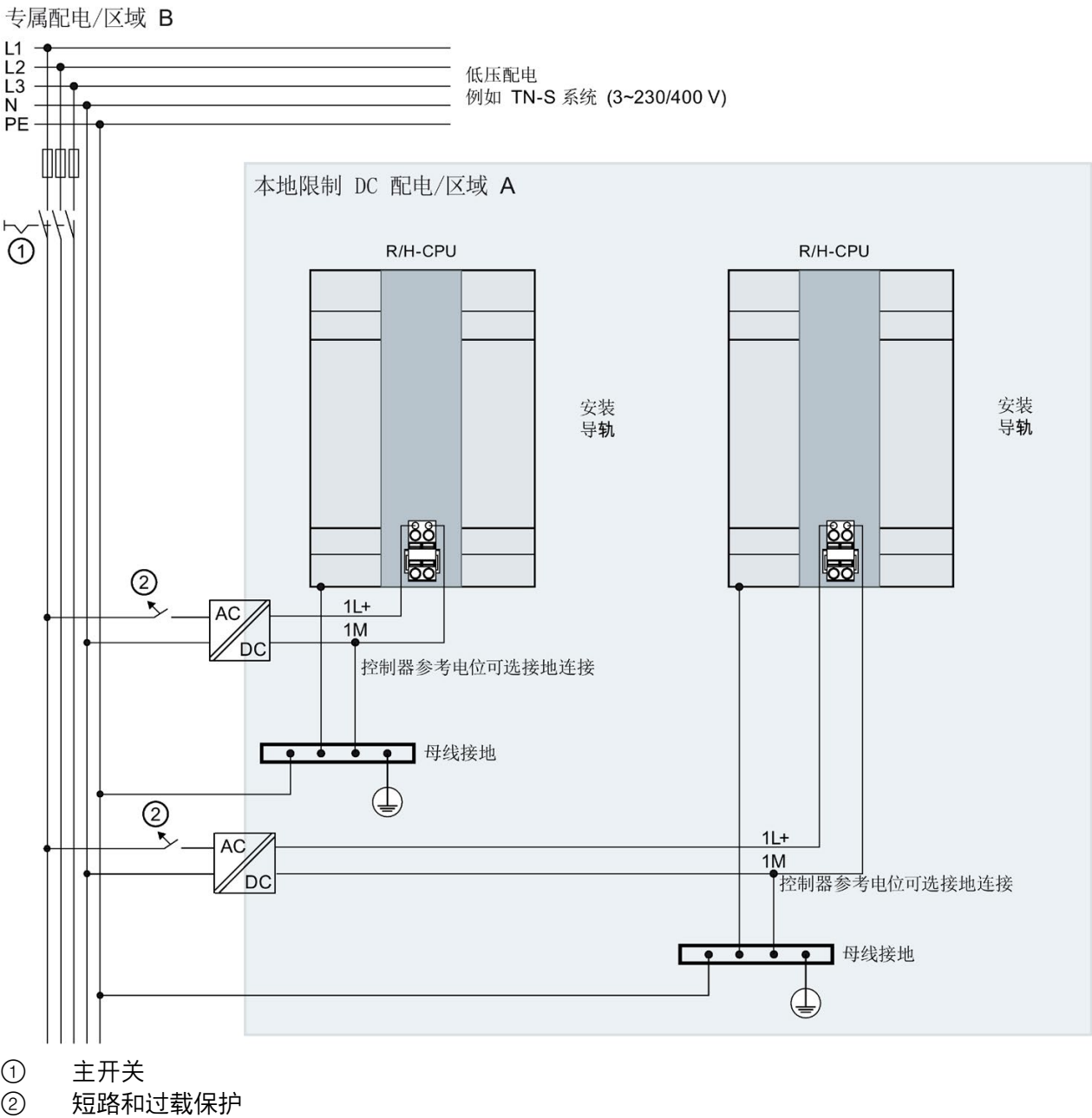
图 7-1 参考电位接地时运行 S7-1500R/H
