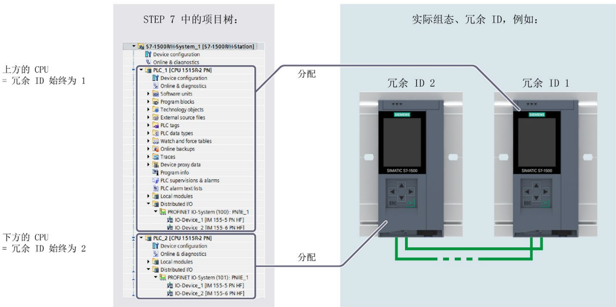
图 11-2 在项目树与实际组态之间分配冗余 ID
