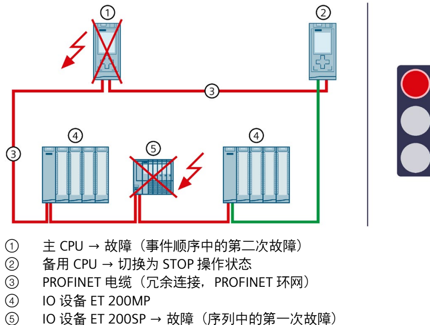
图 5-40 PROFINET 环网中的 IO 设备以及主 CPU 发生故障（以 S7-1500R 为例）
