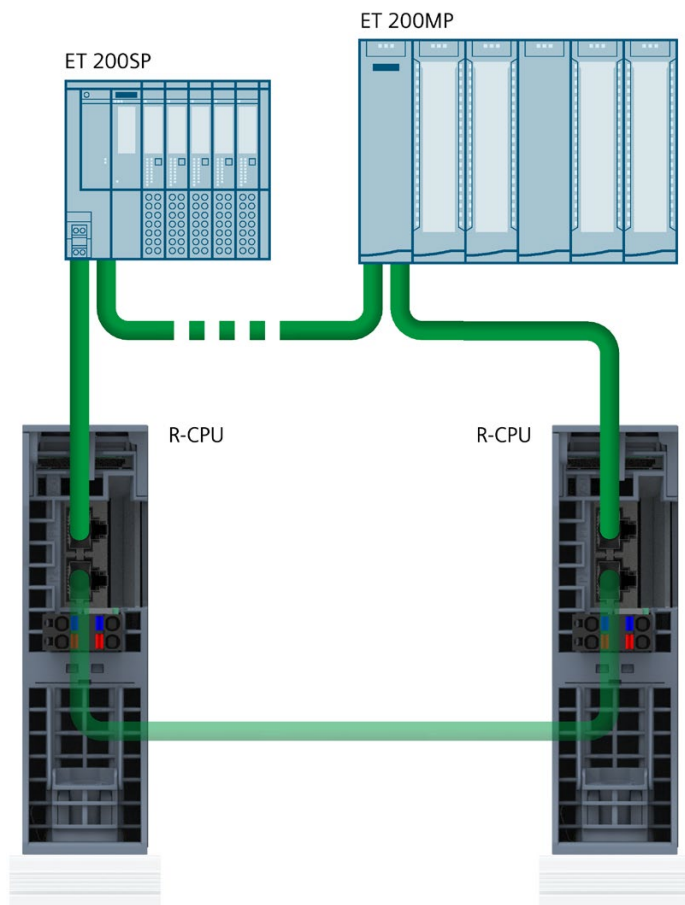
图 7-7 PROFINET 接口 X1 P1R :
