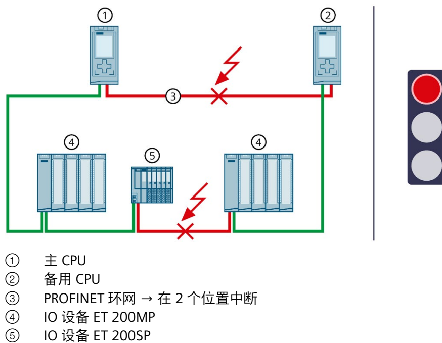
图 5-39 PROFINET 环网中有 2 处电缆中断（间隔不超过 1500 ms）
