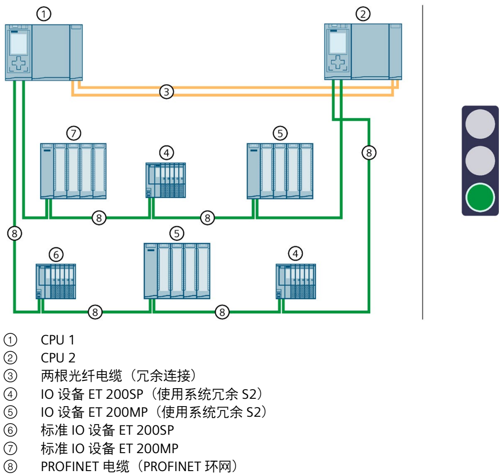
图 5-3 PROFINET 环网中连接了 IO 设备的 S7-1500H 组态
