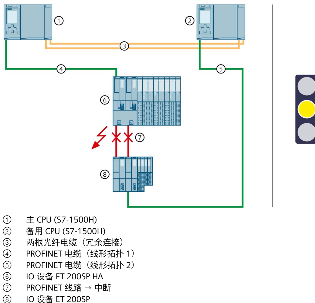
图 5-33 线型拓扑中两个 R1 设备之间的两条 PROFINET 线路故障
