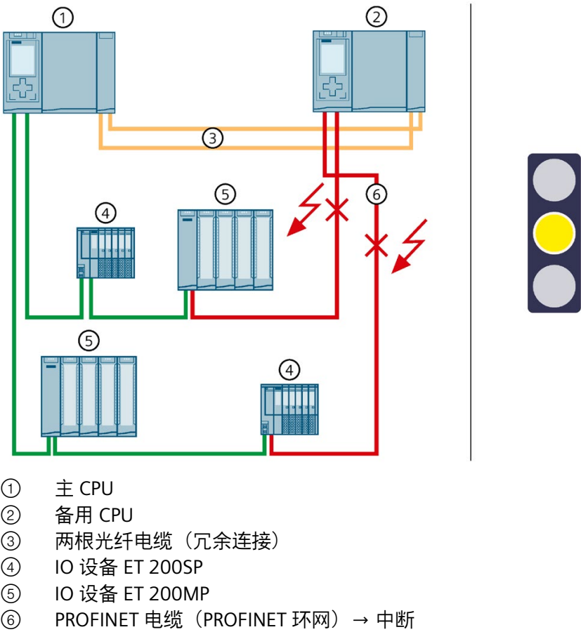
图 5-30 备用 CPU 的 PROFINET 环网中的两根 PROFINET 电缆故障
