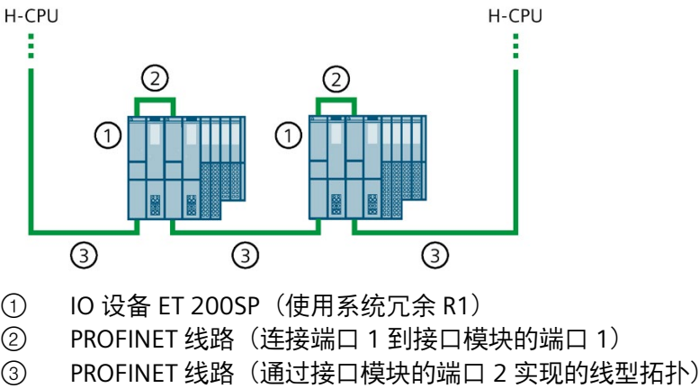
图 5-14 不推荐的组态变型
