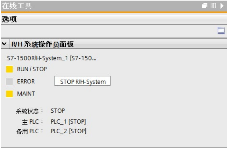
图 11-13 R/H 系统操作面板上的 STOP 系统
