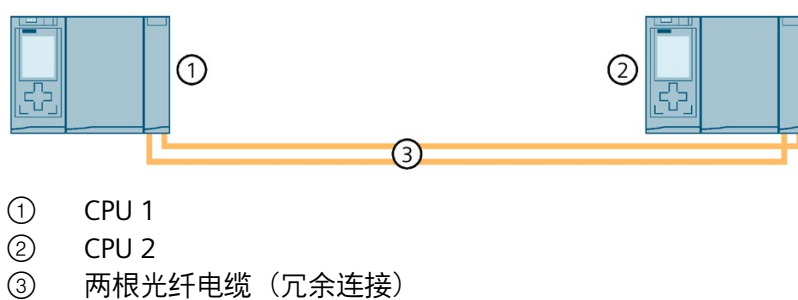
图 5-22 不含附加设备的 S7-1500H 组态
