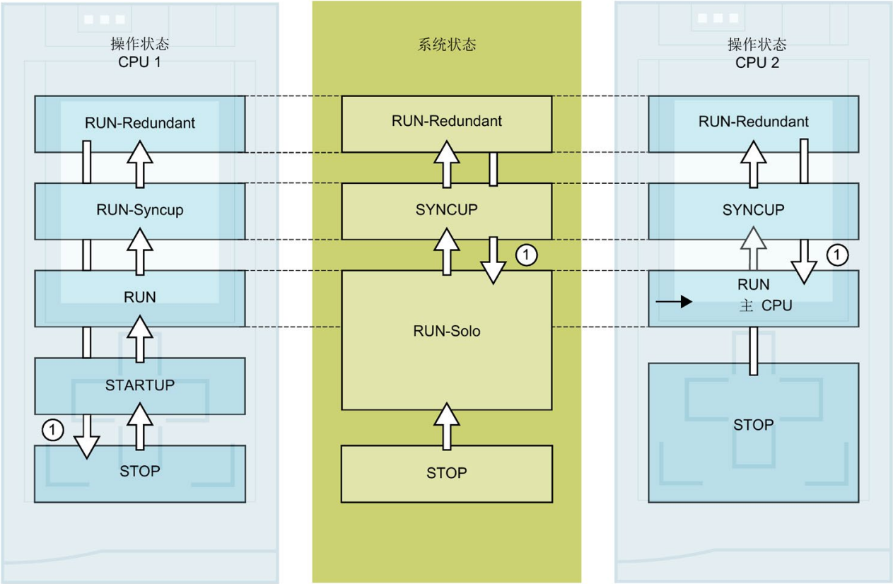
图 11-12 主-备份切换
