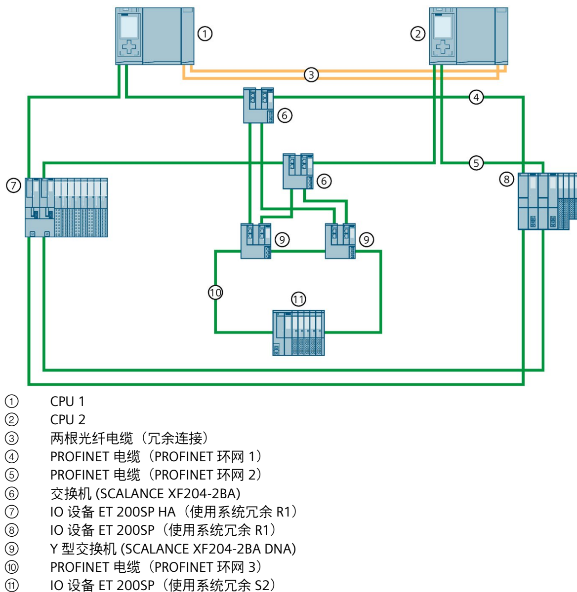
图 5-12 PROFINET 环网中包含 R1 设备和 Y 型交换机（采用 DNA 冗余）的 S7-1500H 组态
