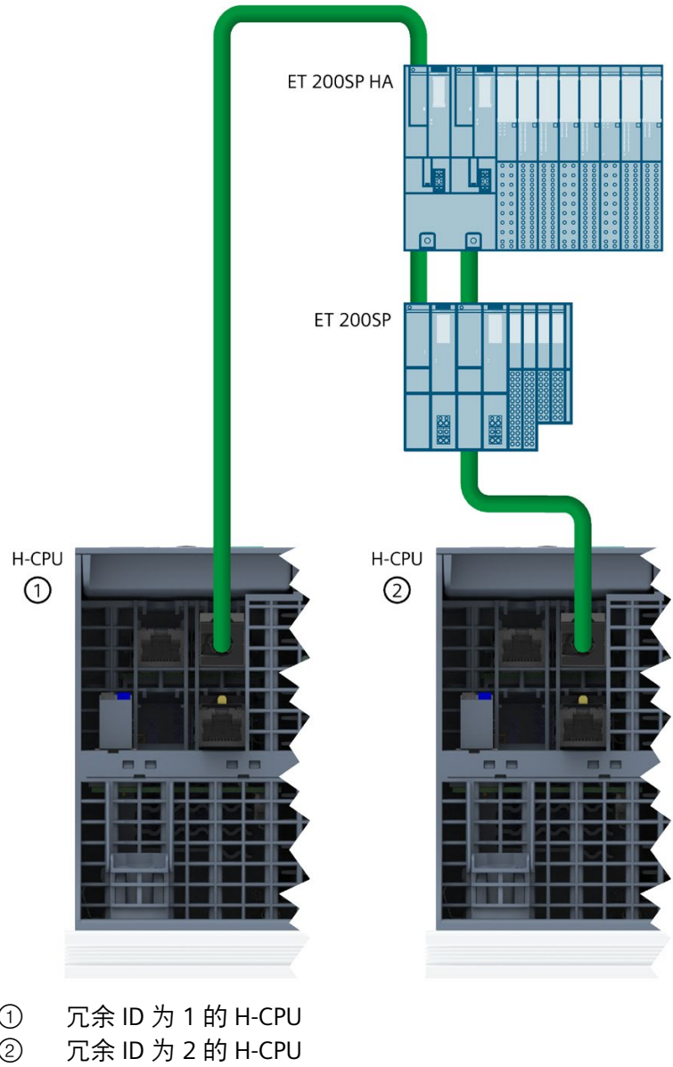
图 7-16 将包含 R1 设备的线型拓扑连接到 S7-1500H
