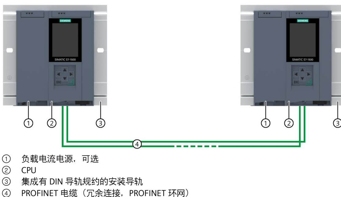
图 4-14 S7-1500R 组态示例
