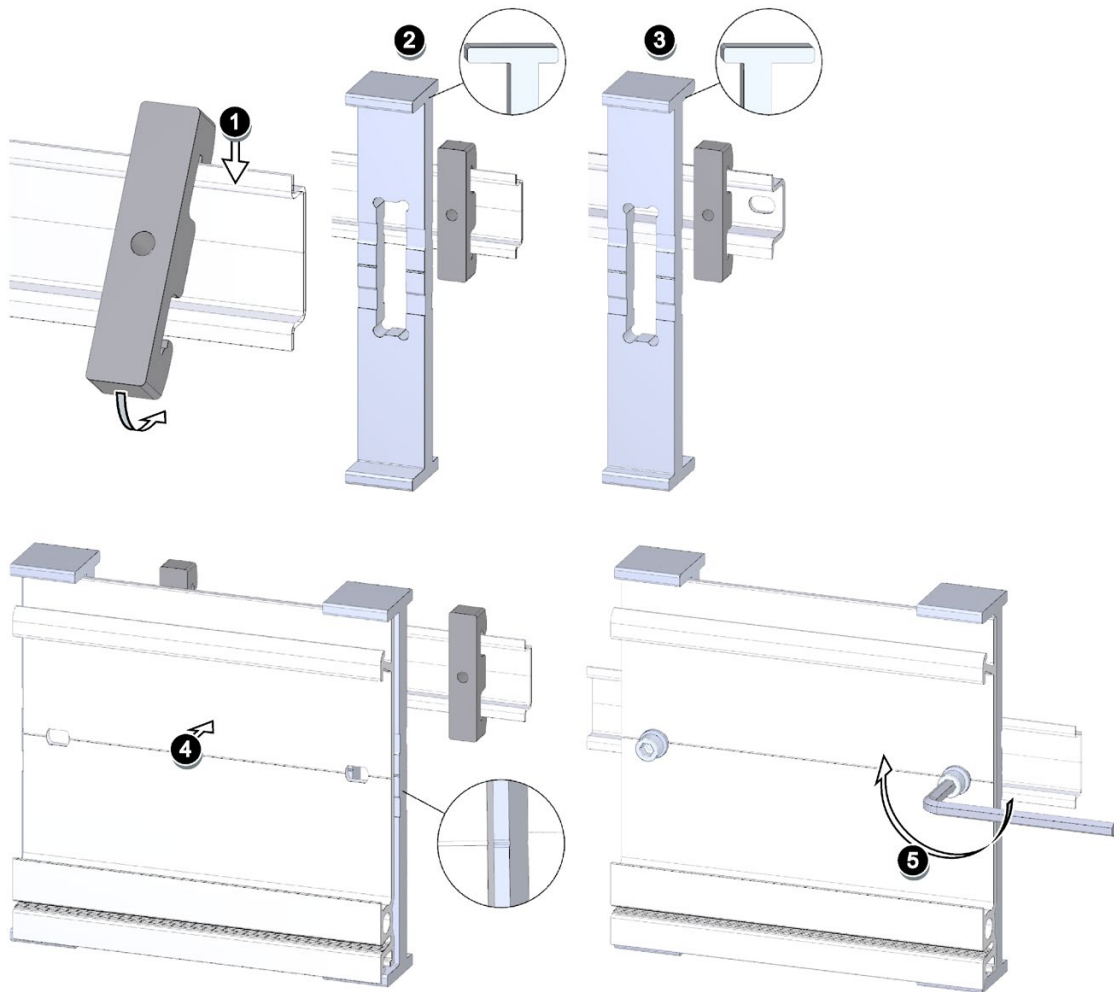
图 6-8 将 DIN 导轨适配器安装到 DIN 导轨 35 mm x 7.5 mm 或 35 mm x 15 mm 的顺序
