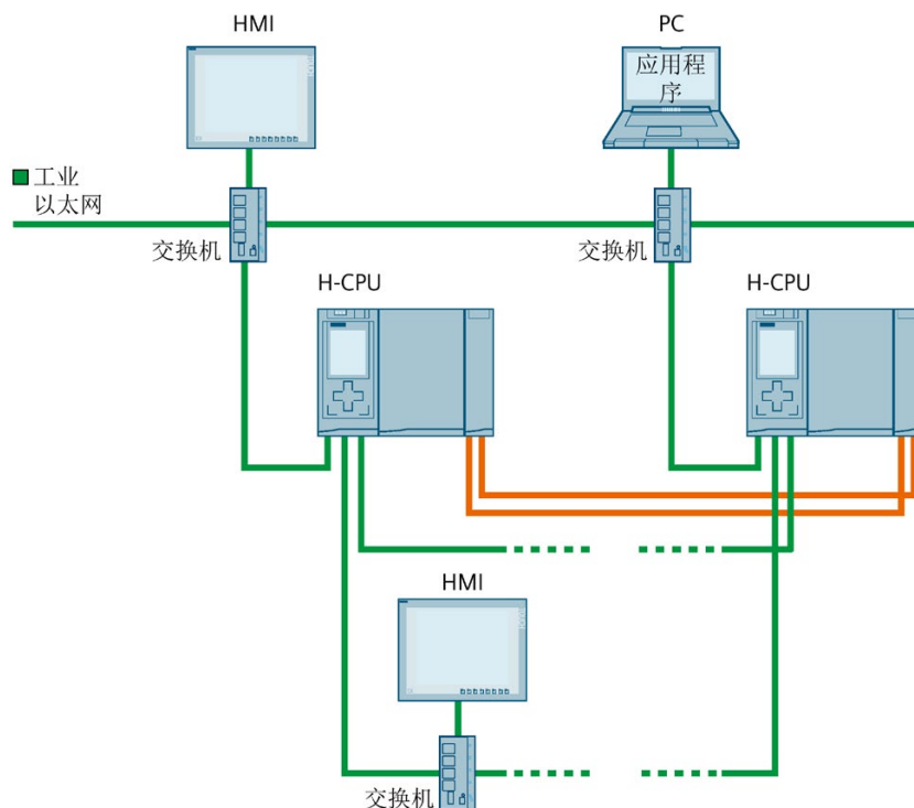
图 5-49 CPU 1518HF-4 PN 组装示例：通过工业以太网和 PROFINET 环网连接 HMI 设备
