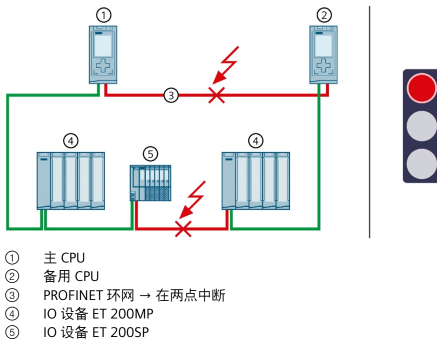
图 5-38 PROFINET 环网中有两处电缆中断（间隔大于 1500 ms）
