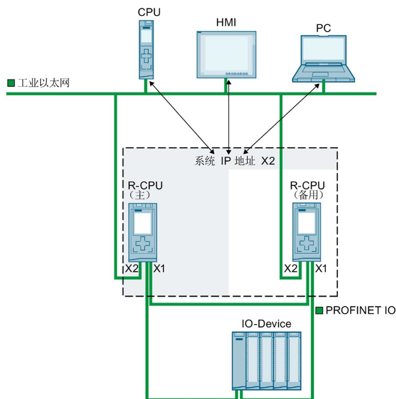
图 4-26 示例：S7 1500R/H 冗余系统通过系统 IP 地址 X2 进行通信
