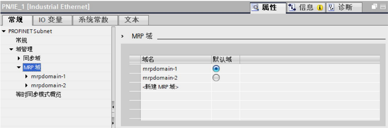
图 8-8 创建另一个 MRP 域“mrpdomain-2”
