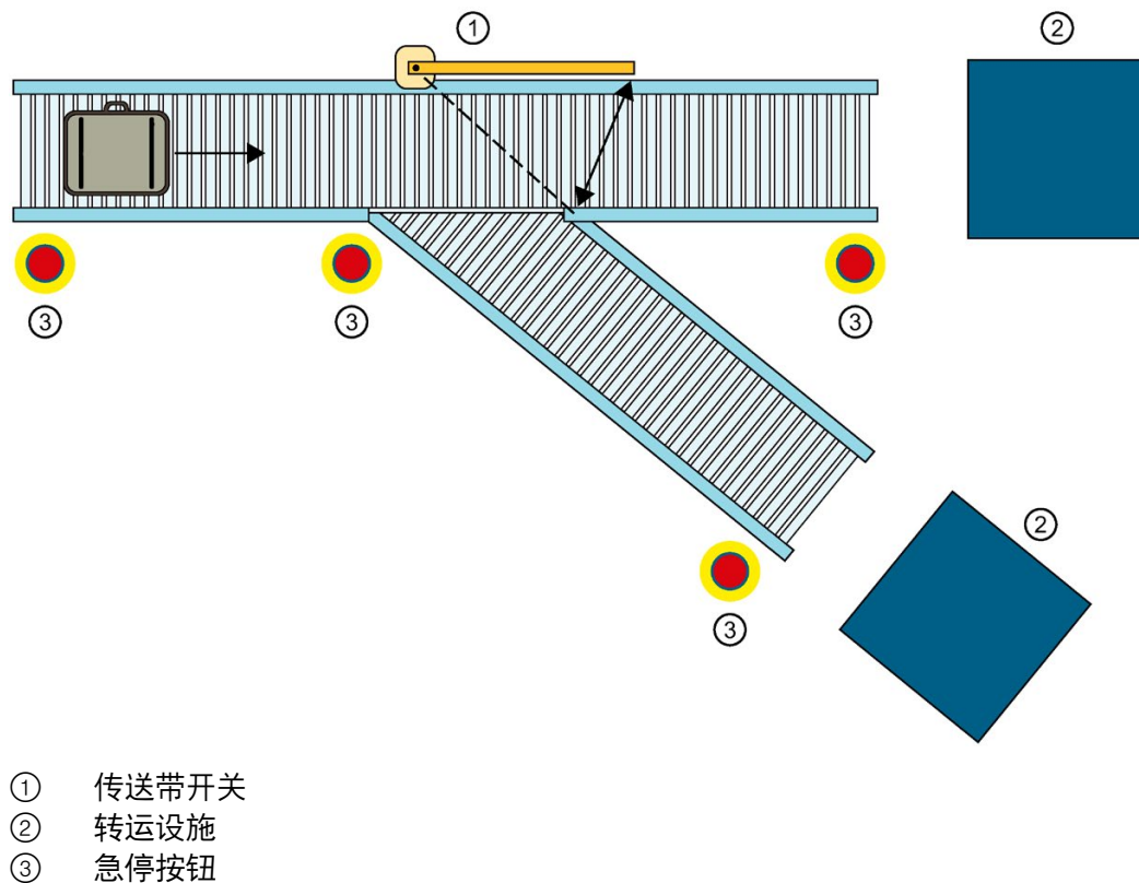
图 4-19 带急停按钮的行李输送系统
