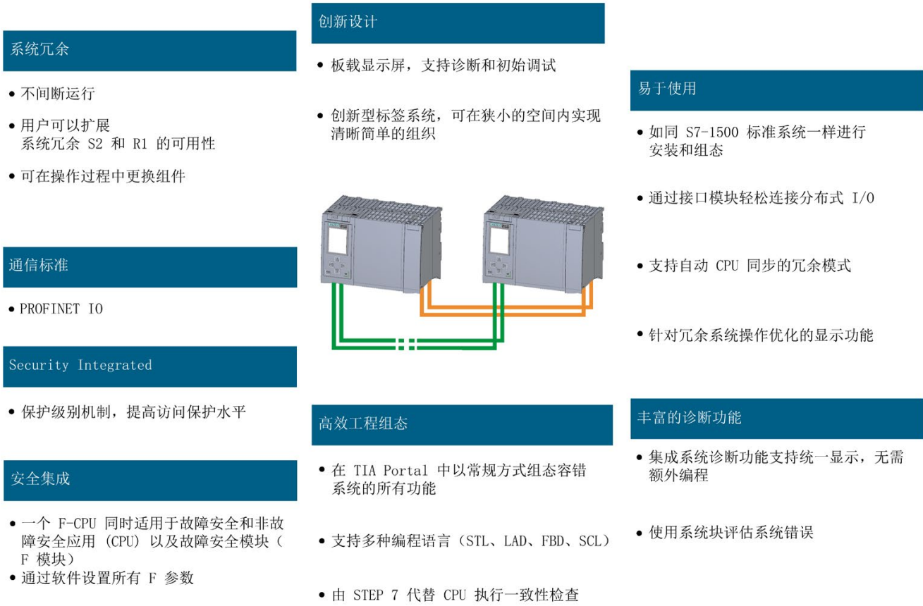
图 4-13 S7-1500R/H 特点
