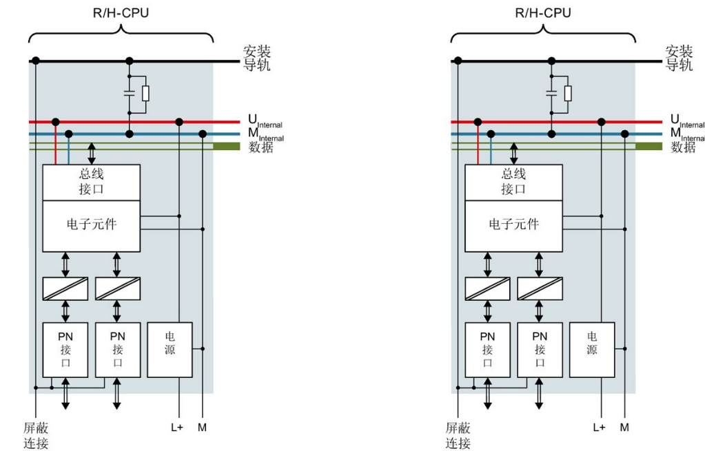
图 7-2 在 CPU 1515R-2 PN 示例中，S7-1500R/H 的相应电位
