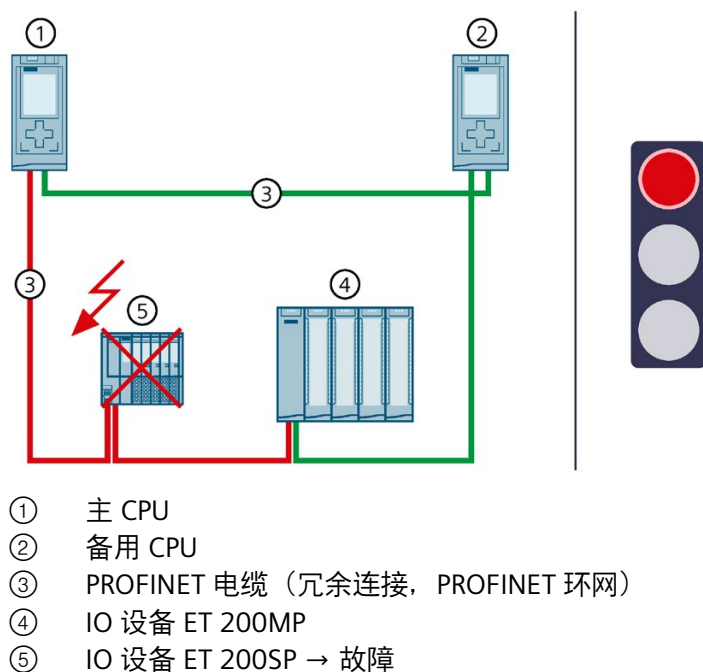
图 5-36 PROFINET 环网中的 IO 设备发生故障（以 S7-1500R 为例）
