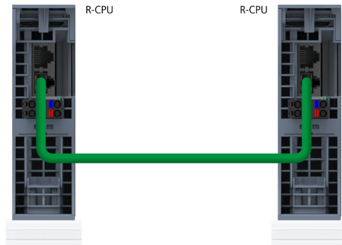
图 7-6 PROFINET 接口 X1 P2R：连接 R-CPU（仰视图）
