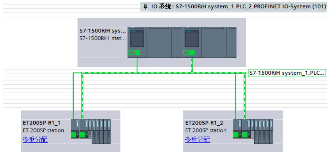
图 8-10 采用系统冗余的网络视图中分配的 R1 设备
