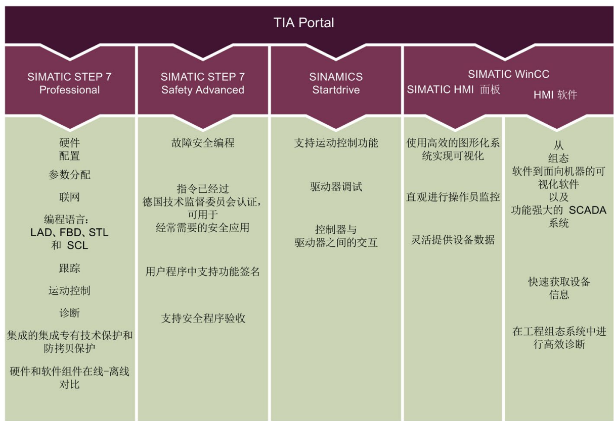
图 4-27 TIA Portal 概述
