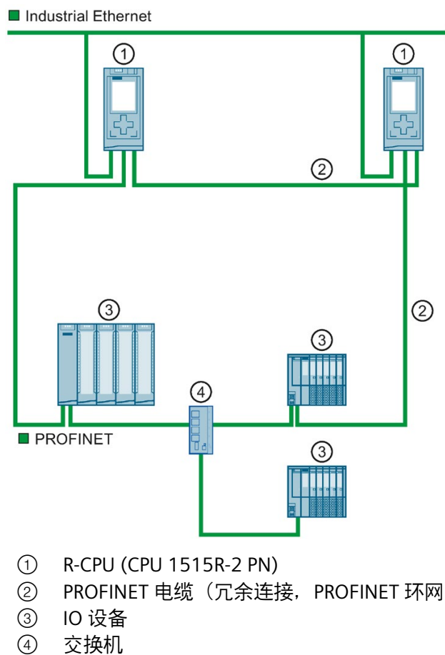
图 4-4 PROFINET 环网中的 S7-1500R 组态
