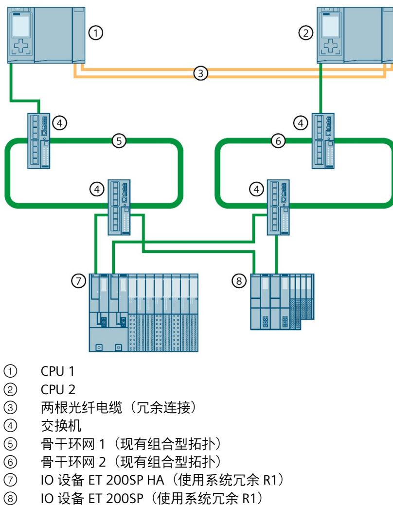
图 5-21 包含 R1 设备和骨干环网的 S7-1500H 组态
