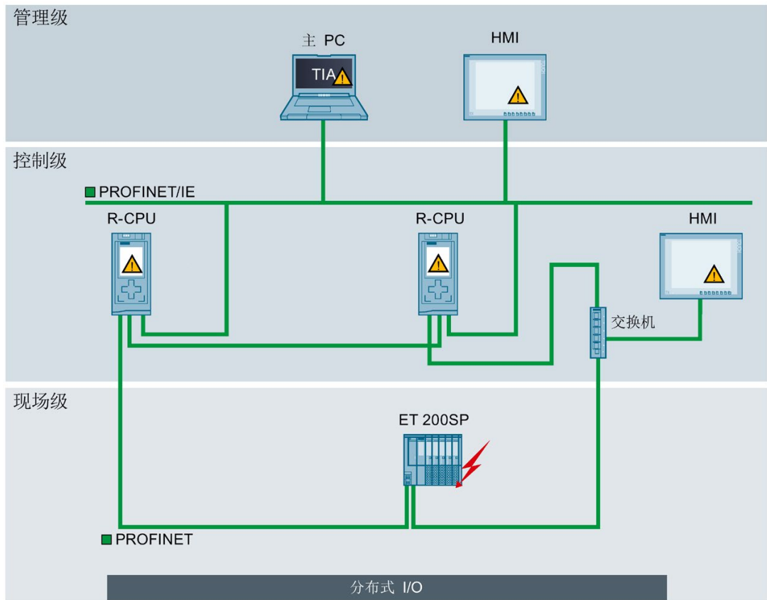
图 4-22 工厂内系统诊断的概述
