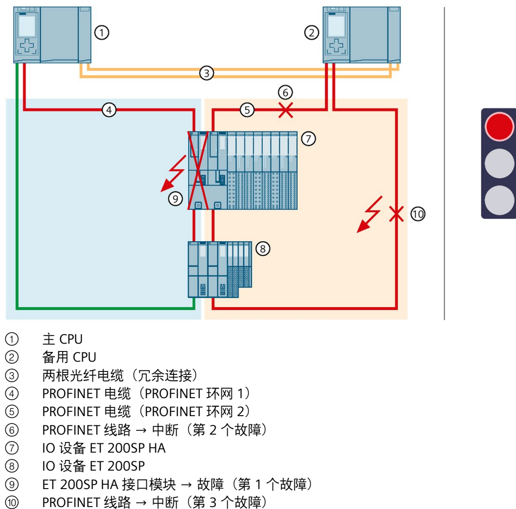
图 5-45 R1 设备中的接口模块和 PROFINET 环网两个位置的 PROFINET 线路出现故障。
