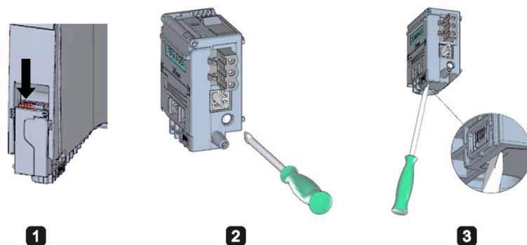
图 7-4 连接电源电压和负载电流电源 (1)
